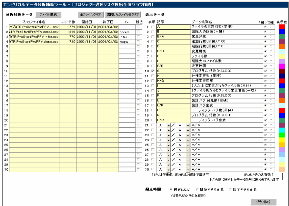
図 6 プロジェクト遅延リスク検出全体グラフ作成画面
